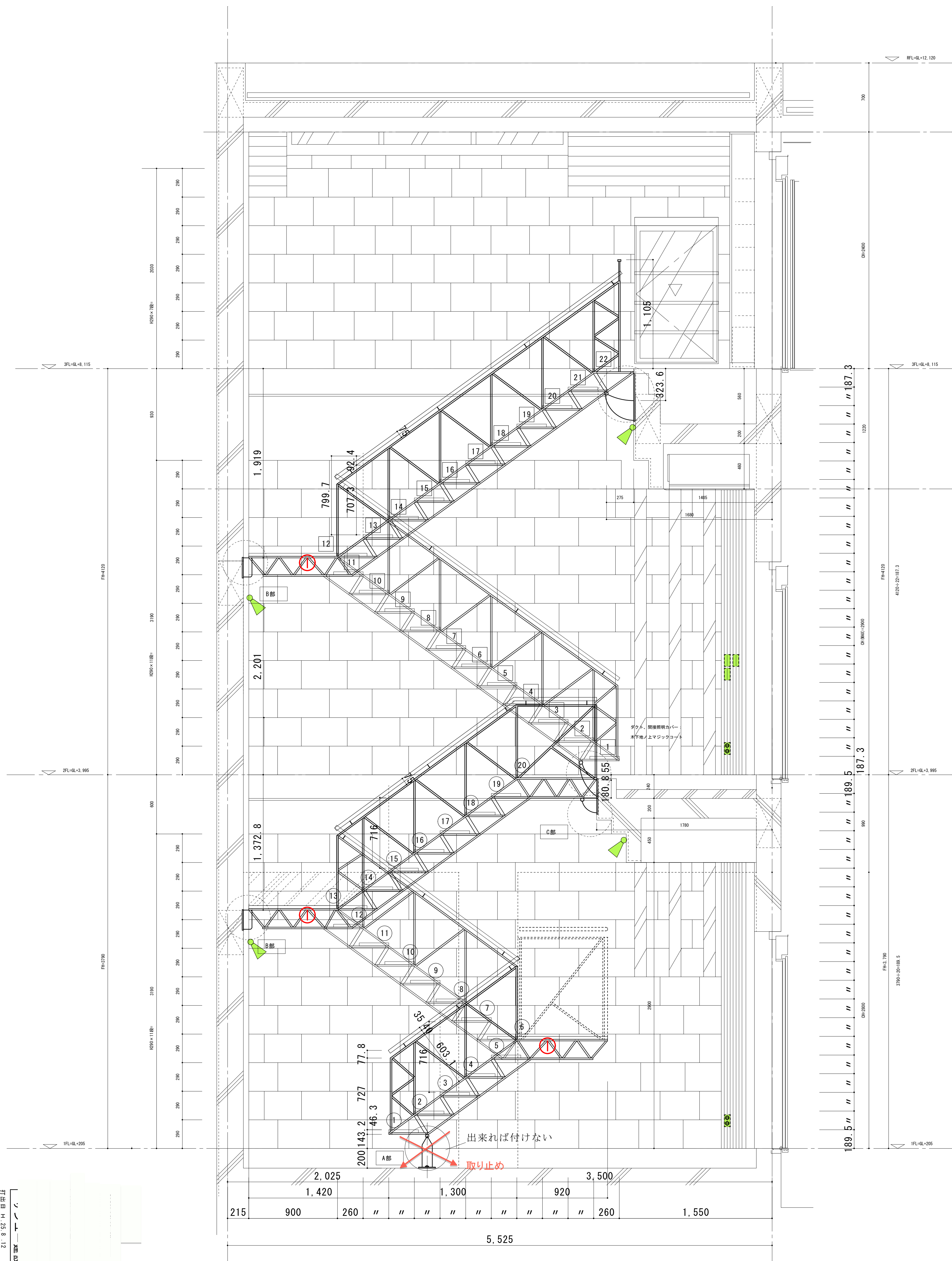
階段断面詳細図 -2 1/20
